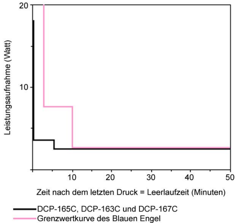
Leistungsaufnahme und Aktivierungszeiten des DCP-165C, DCP-163C und DCP-167C in der Zeit nach dem letzten Druck
