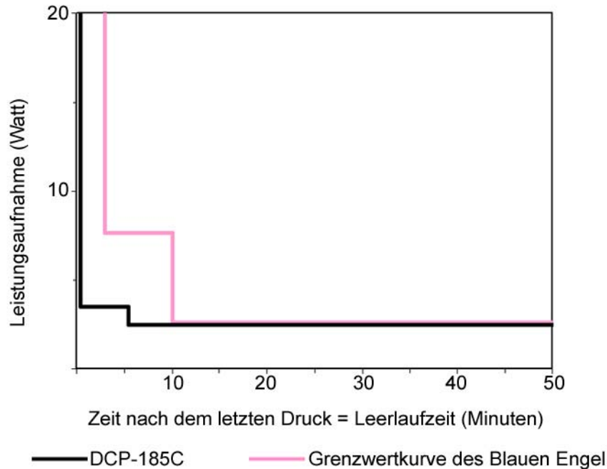
Leistungsaufnahme und Aktivierungszeiten des DCP-185C in der Zeit nach dem letzten Druck
