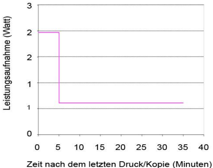
Leistungsaufnahme und Aktivierungszeiten des DCP-J132W in der Zeit nach dem letzten Druck
